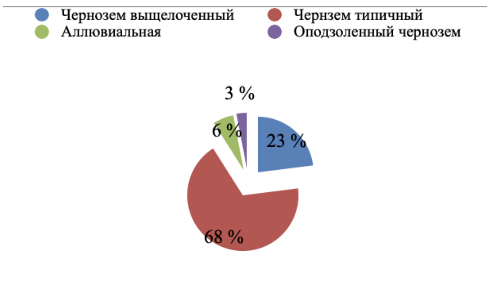
Рисунок 1 - Почвенный покров Донского сельсовета
