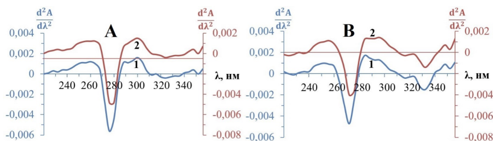
Рисунок 2. Спектральные кривые производных второго порядка катионной (А) и анионной (В) форм ципрофлоксацина.
