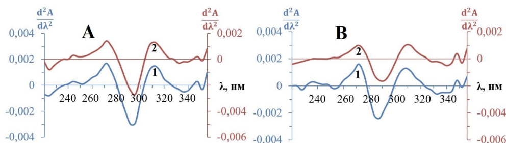
Рисунок 1. Спектральные кривые производных второго порядка катионной (А) и анионной (В) форм офлоксацина.
