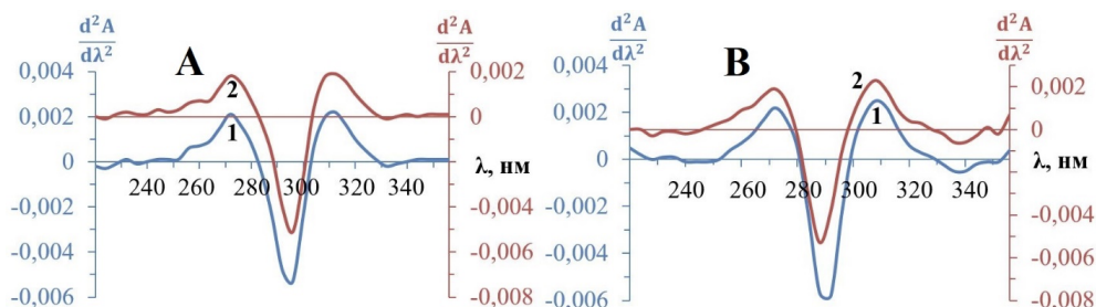
Рисунок 3. Спектральные кривые производных второго порядка катионной (А) и анионной (В) форм моксифлоксацина.
