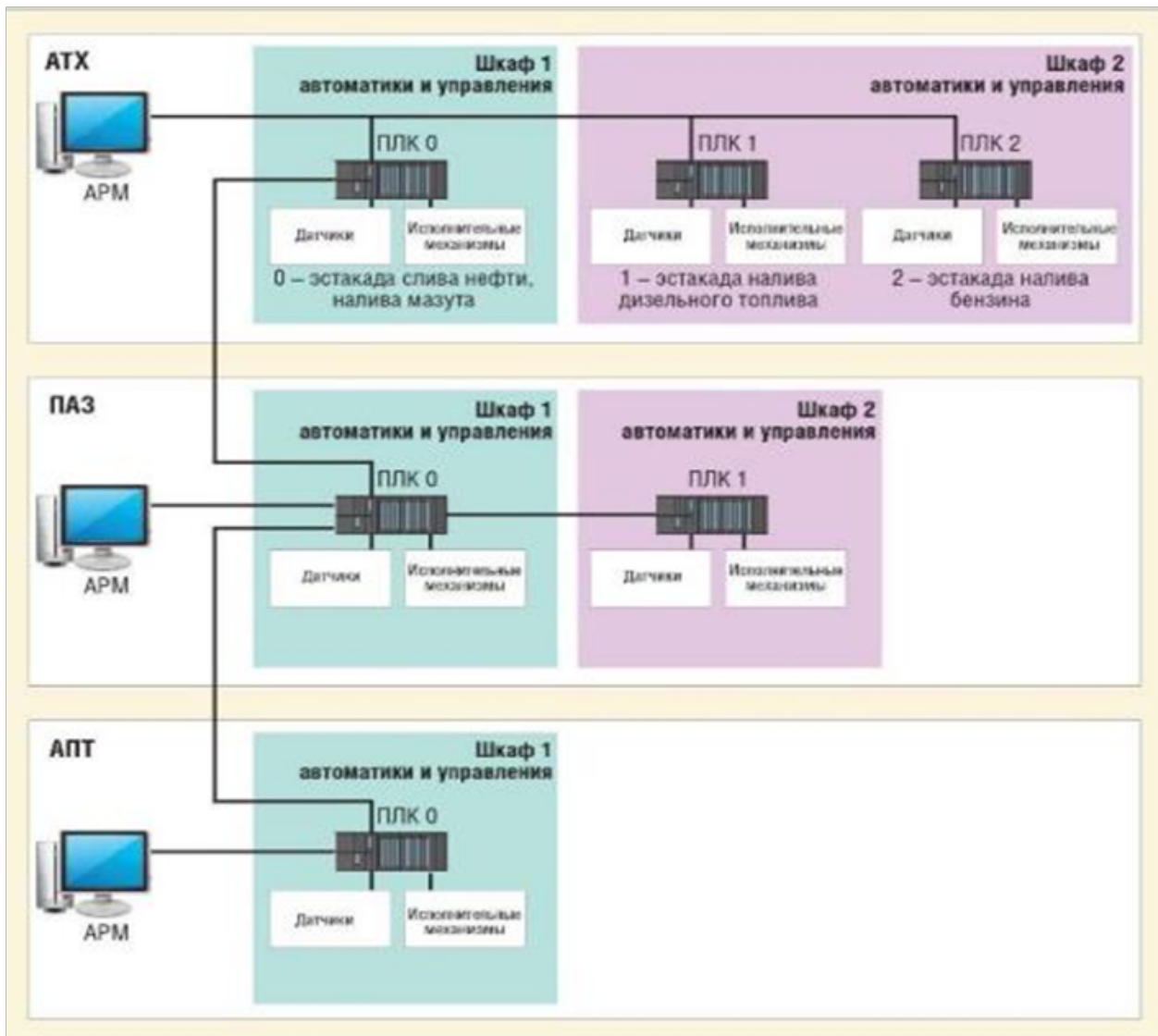
Рисунок 1 - Схема автоматизированной системы управления сливноналивной эстакады
