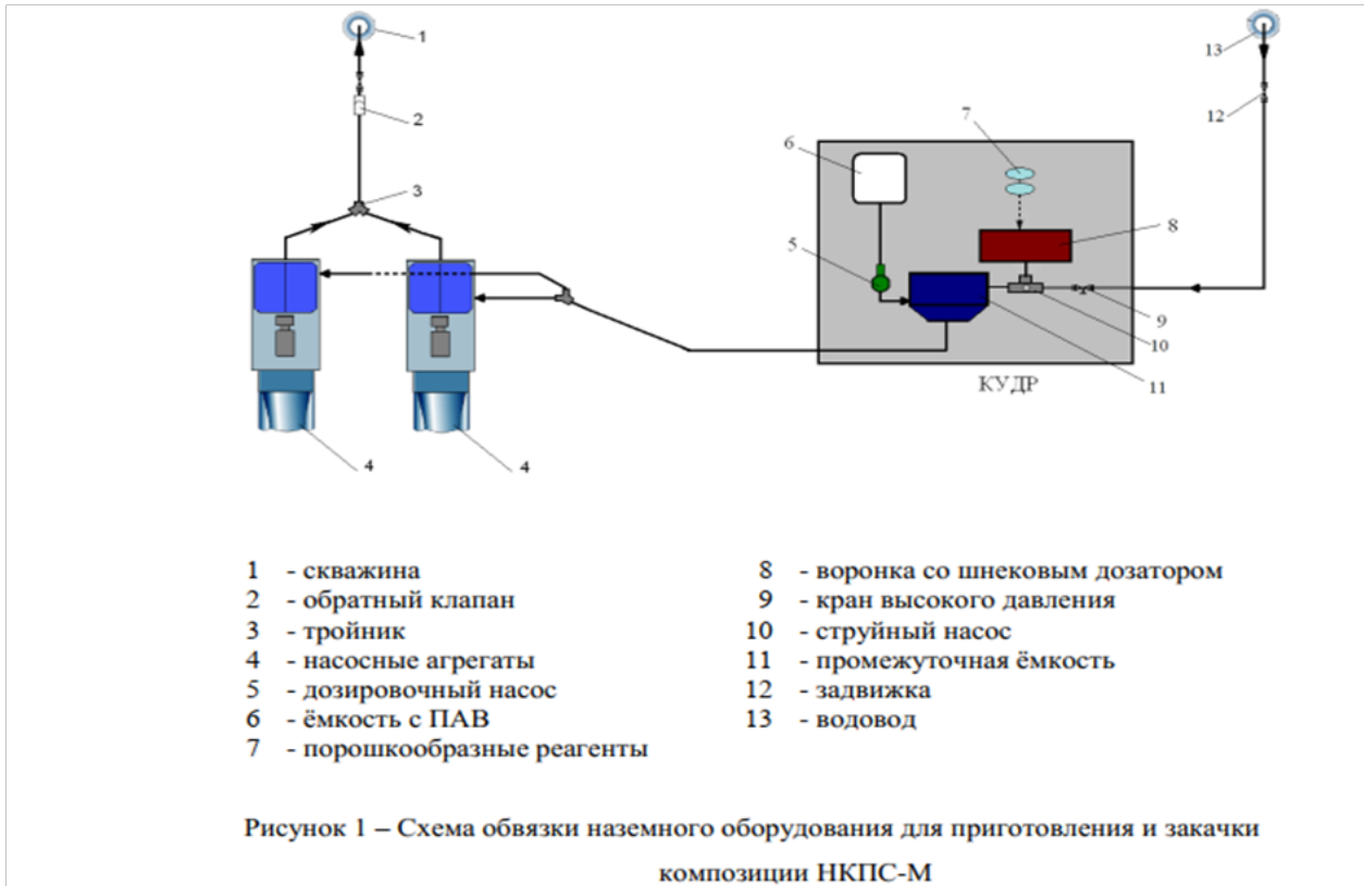
Рисунок 1. Схема обвязки наземного оборудования и устья скважины
