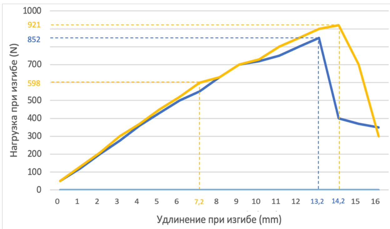
Рис. 5. График среднестатистических показателей образцов без УФ облучения (синий) и с УФ облучением (желтый)
