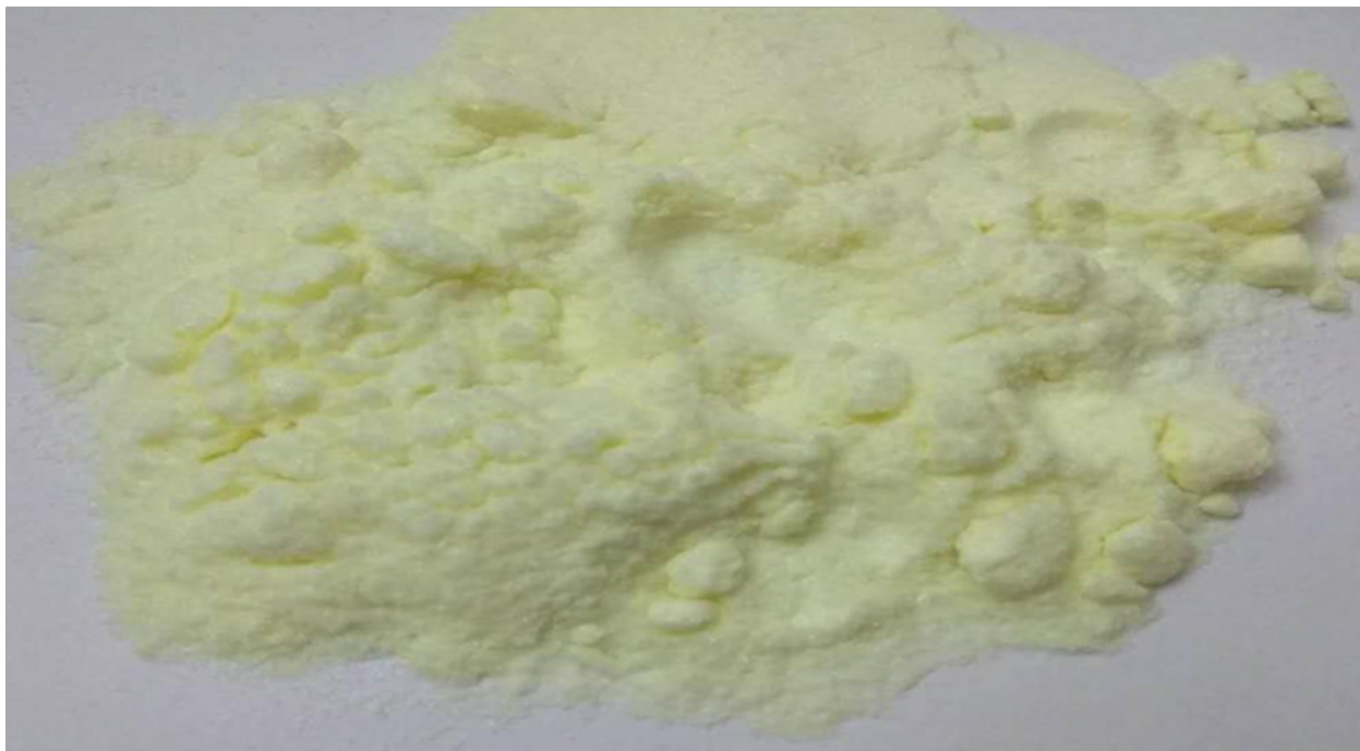
Рис. 1. УФ-стабилизатор UV-531
