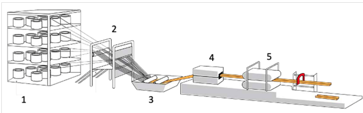
Рис. 2. Производственная установка для формирования образцов однонаправленного стеклопластика;
