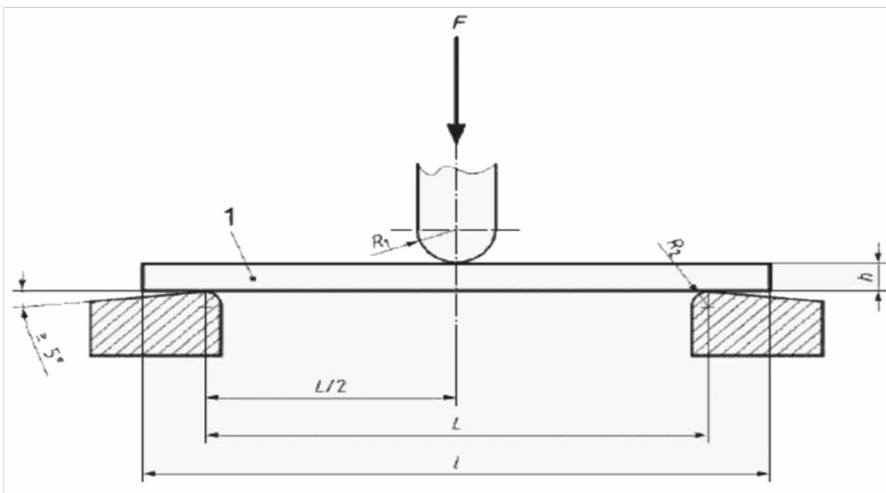
Рис. 4. Схема положения образца в начале испытаний
